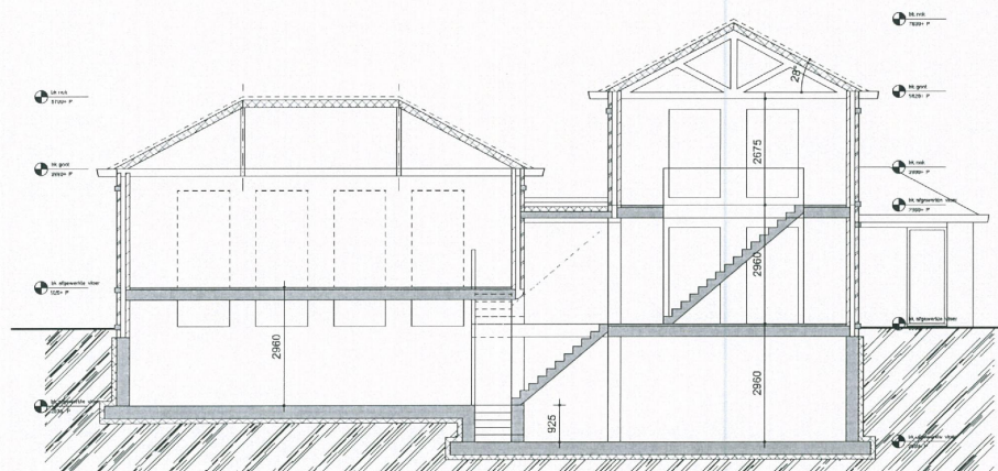
langsdoorsnede (B)
