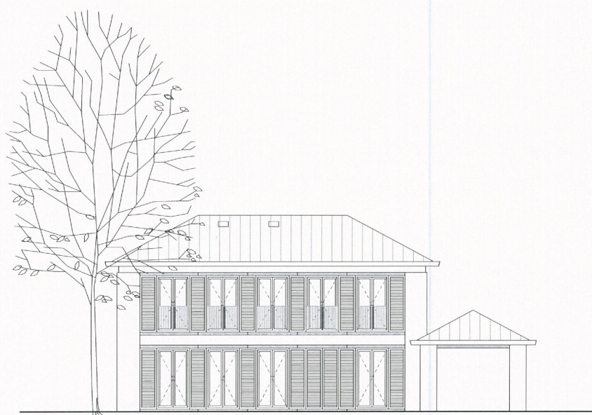
zuidgevel (achtergevel)
